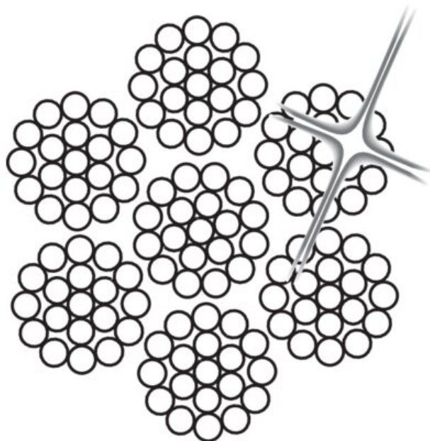
Teräsköysiraksi
